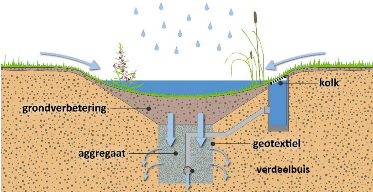
Figuur 20: opbouw van een wadi (blaugroenvlaanderen)
